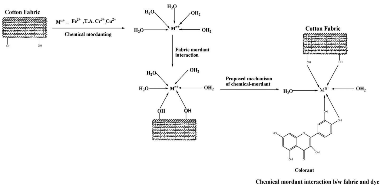
ภาพที่ 3 กลไกการย้อมติดของมอร์แดนต์ยางกล้วยน้ำว้าผ่านพันธะไฮโดรเจน
